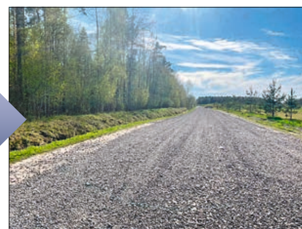
Отсыпка щебнем подъездной дороги
