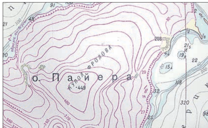
Ледник Фролова на острове Пайера в арх. Земля Франца-Иосифа
